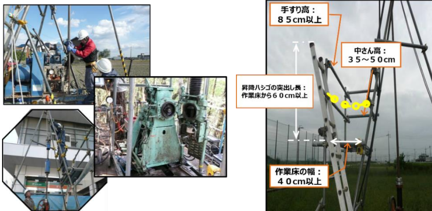
高所作業床（安全ヤグラ） 設置状況
