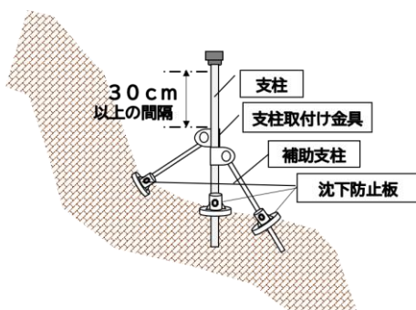
モノレール支柱（斜め支柱）の取付例
