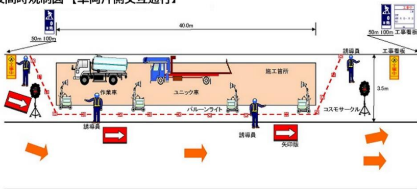
夜間時規制図【車両片側交互通行】
