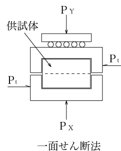
一面せん断法
