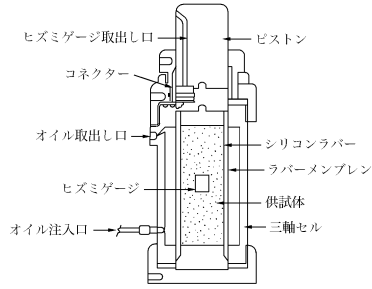
三軸セル
