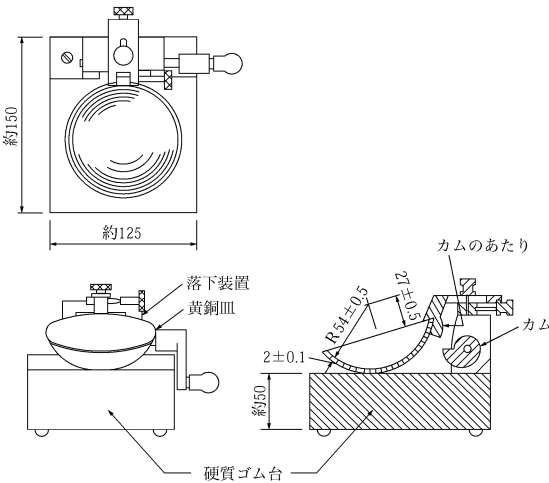
液性限界測定器 (単位: mm)
