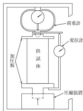
ひずみ制御式一軸圧縮試験機の例
