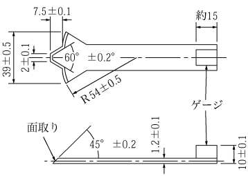
溝切りおよびゲージ (単位: mm)
