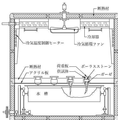
凍上試験キャビネット概念図
