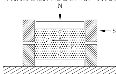
一面せん断試験概念図
