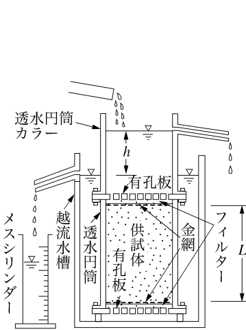
定水位透水試験の概念図
