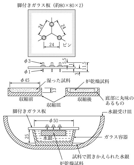
収縮定数試験用具の例 (単位: mm)
