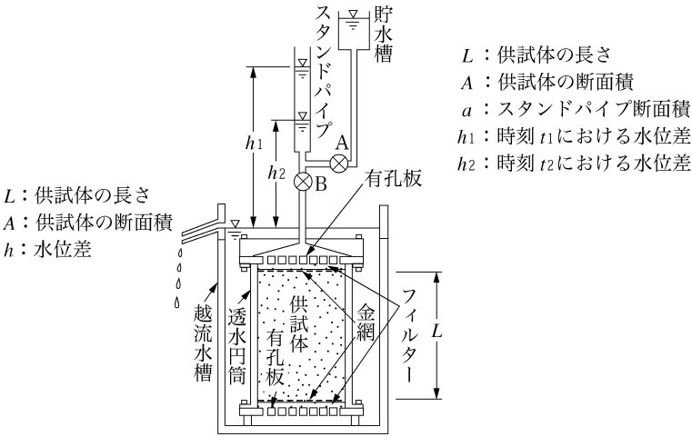
変水位透水試験の概念図
