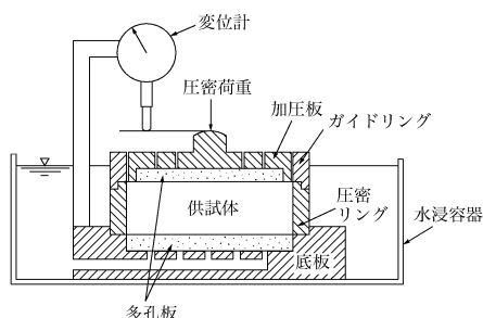
圧密容器のご概念図
