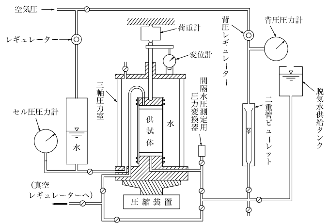
三軸試験機の構成例
