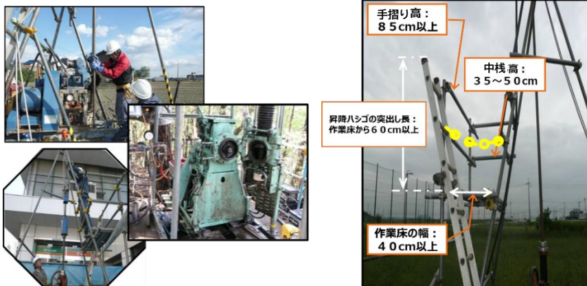
ボーリング作業状況
