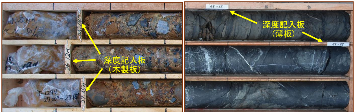
写真 10-4 深度記入板の例
