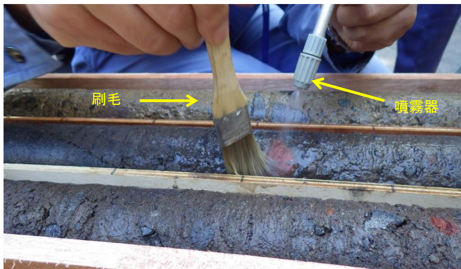
写真 10-10 噴霧器と刷毛を使った洗浄 (軟質部を流失しないよう注意する。)
