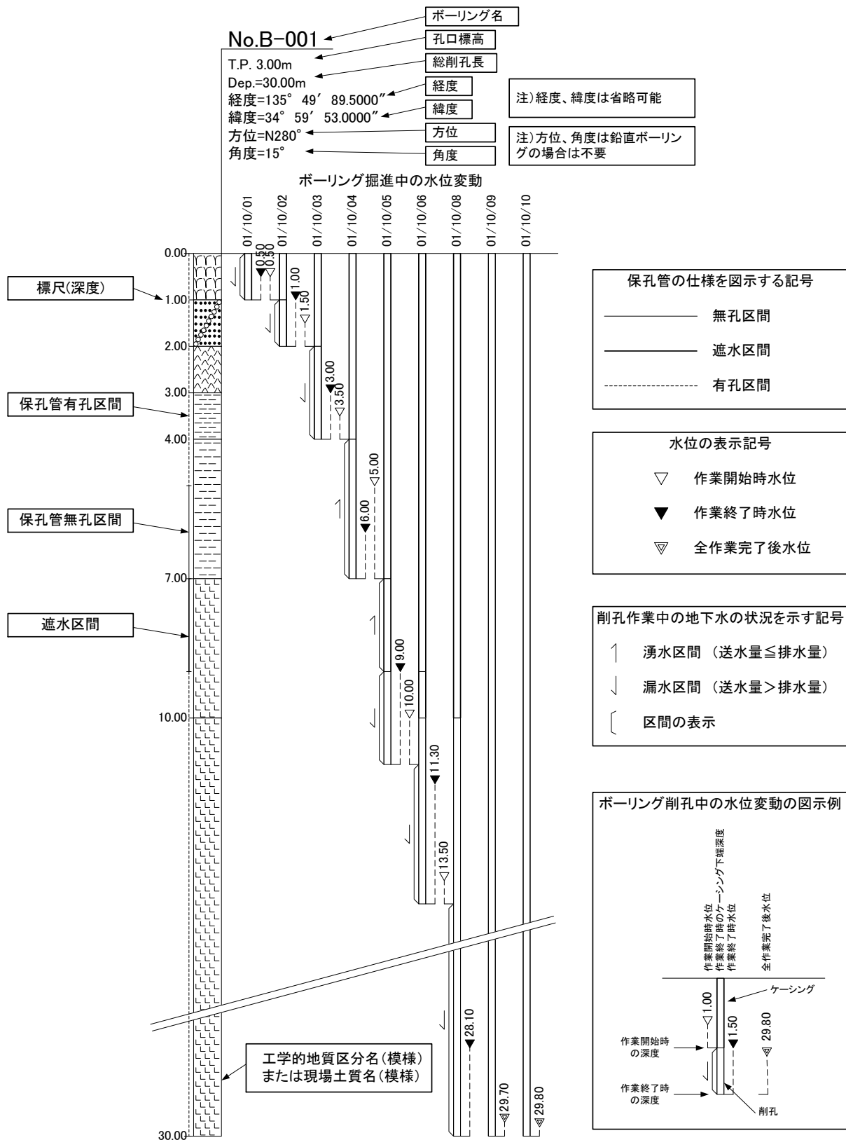
図 7-3 ボーリング掘進中における水位変動の記載例
