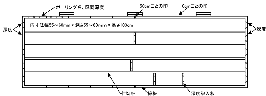
図 10-1 コア箱記入例
