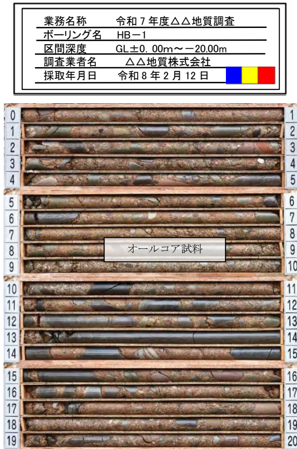
図 8-4 連続ボーリングコア写真の整理例 (2)
