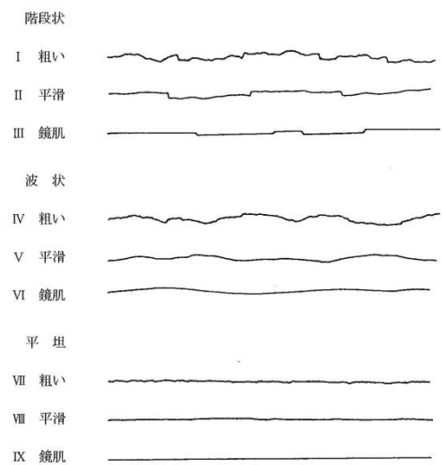
図 3-2 不連続面の粗さのカテゴリの代表断面（IAEG 2) を翻訳）
