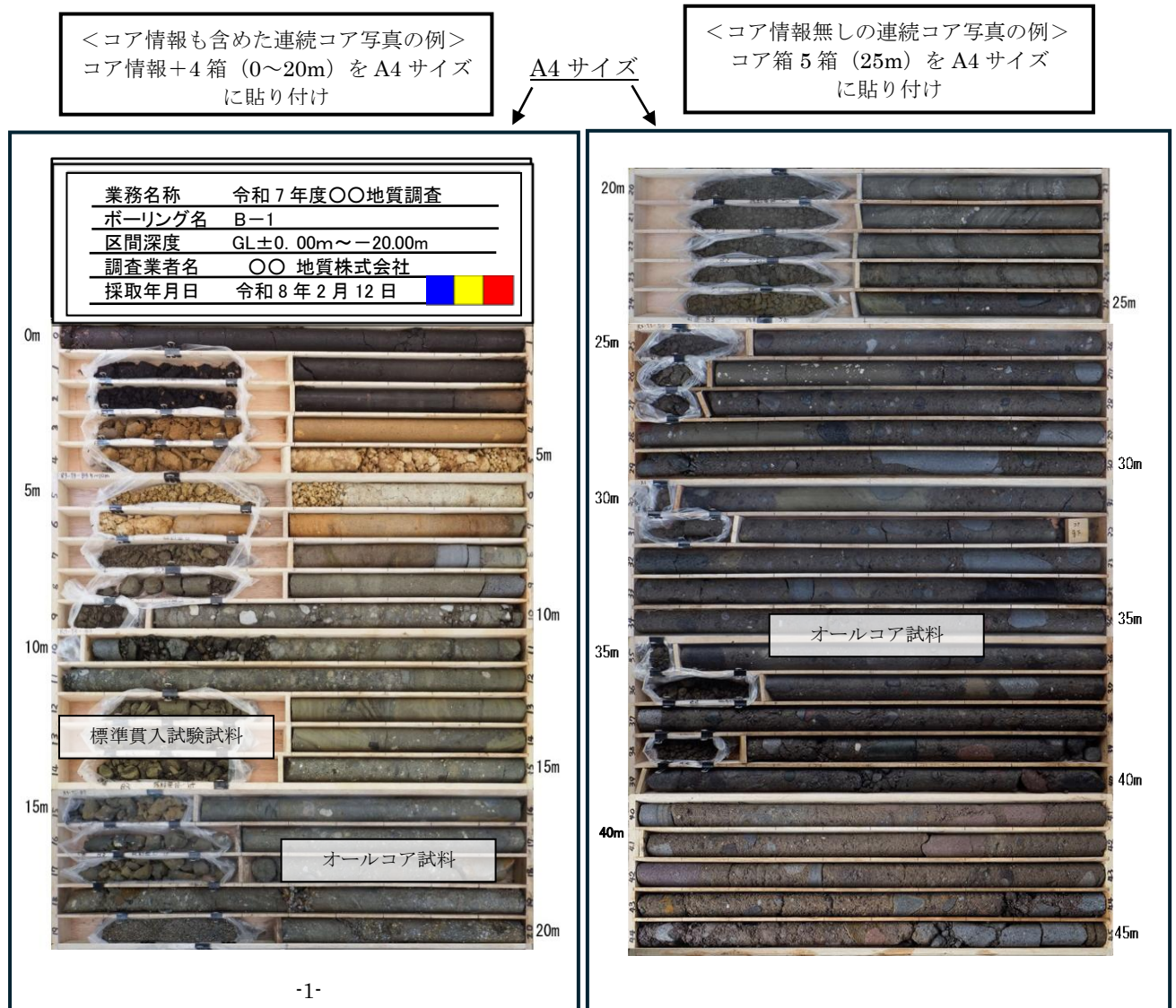
図 8-3 連続ボーリングコア写真の整理例(1)
