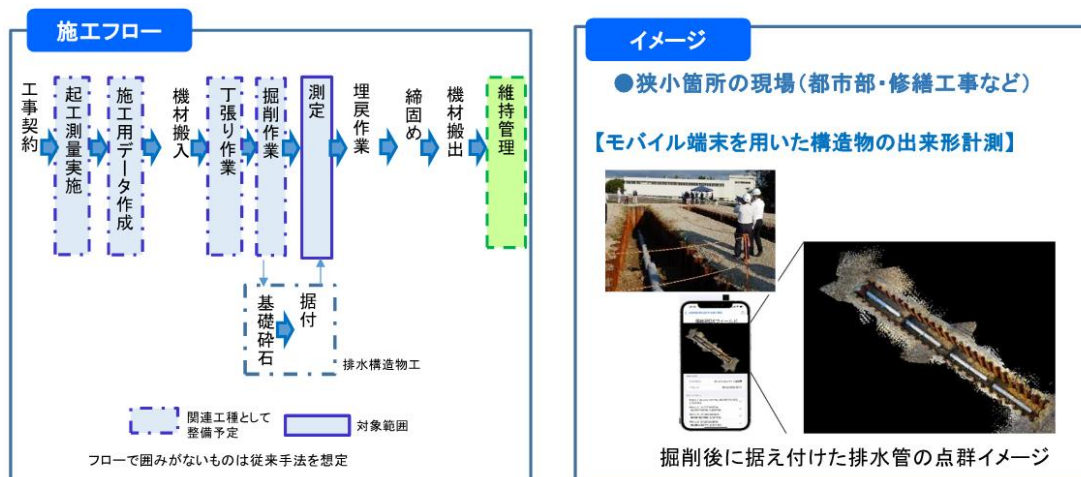
図 5-10 小規模現場への ICT 適用拡大:モバイル端末を用いた構造物の出来形計測
