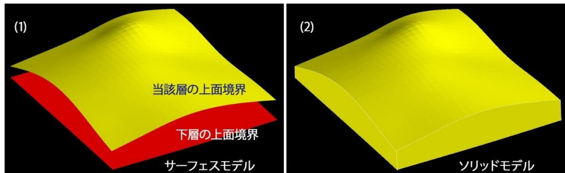
図 6-9 ソリッドモデル (B-reps) の例
