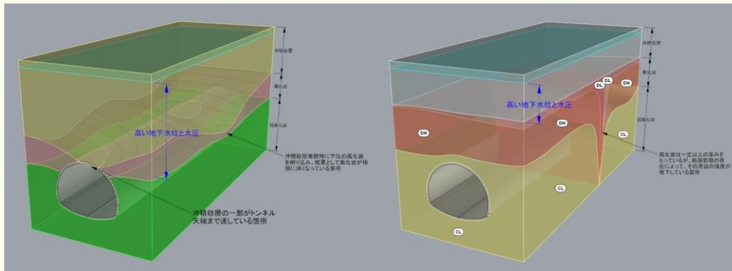
図 4-12 トンネルの地質リスクの可視化 (例)
