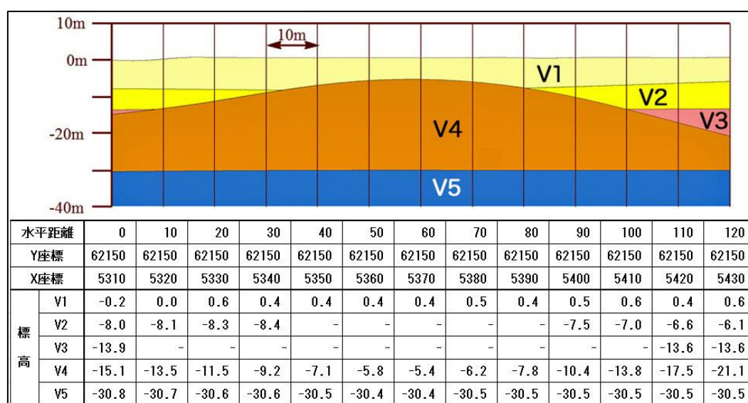
図 6-11 パネルダイアグラムの例
