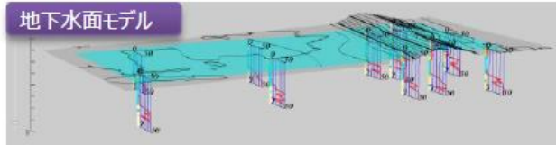
図 4-9 目的に応じたモデルの作成例
