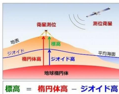
図 2-4 楕円体高、ジオイド高、標高の関係
