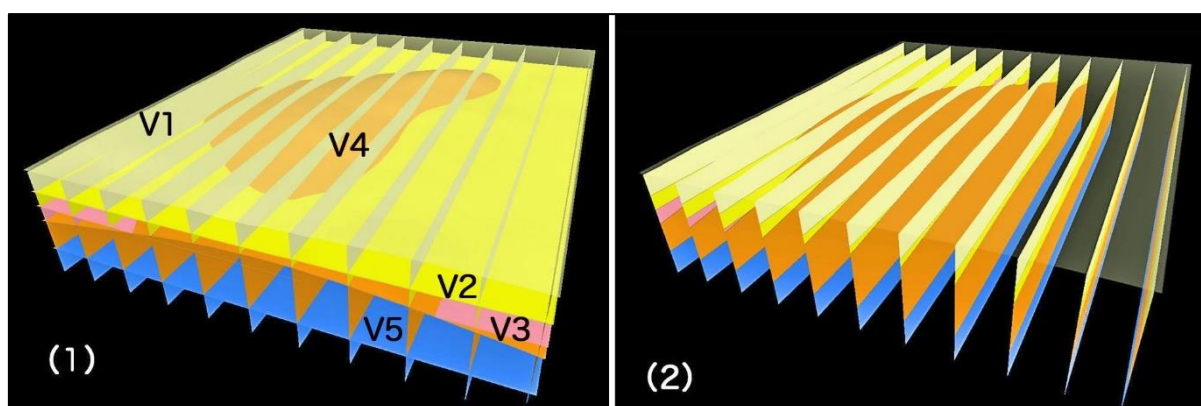
(左) サーフェスモデル＋パネルダイアグラム (右) 地表面＋パネルダイアグラム
