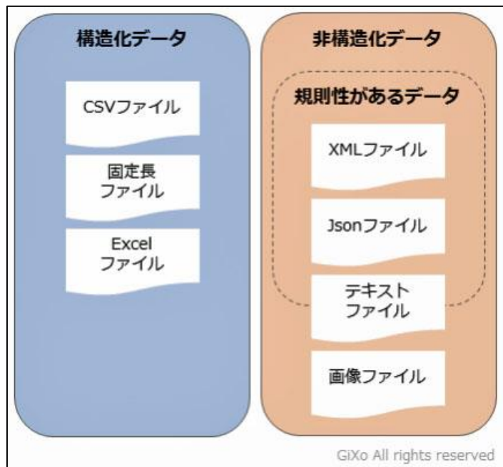
図 1-5 構造化データと非構造化データ
