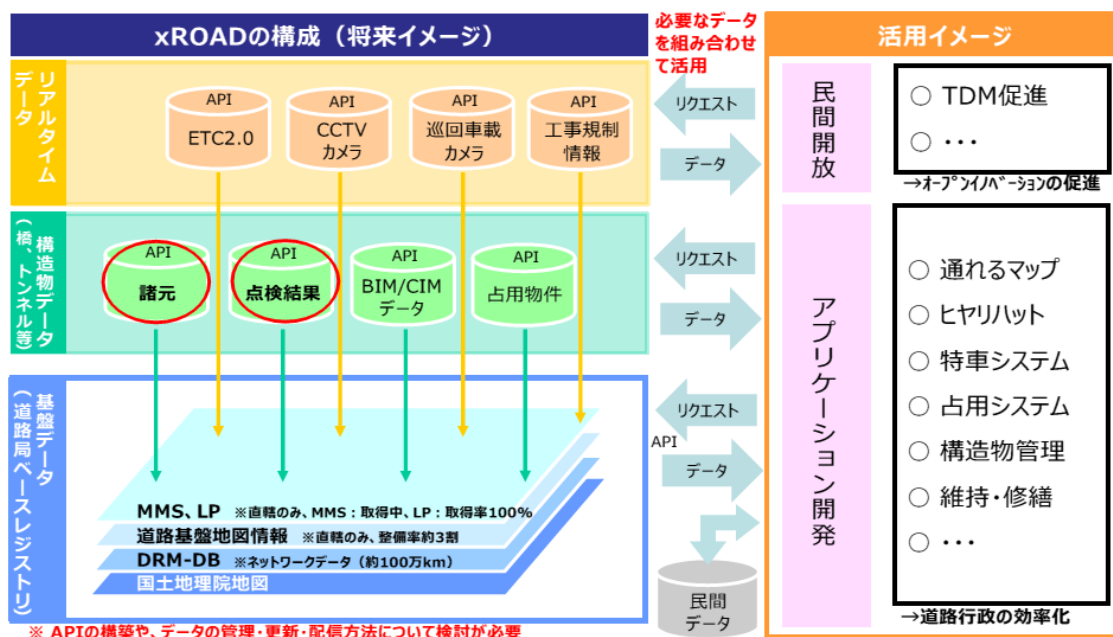
図 5-29 xROAD（道路データプラットフォーム）の構成
