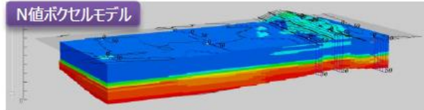
地下水面モデル
