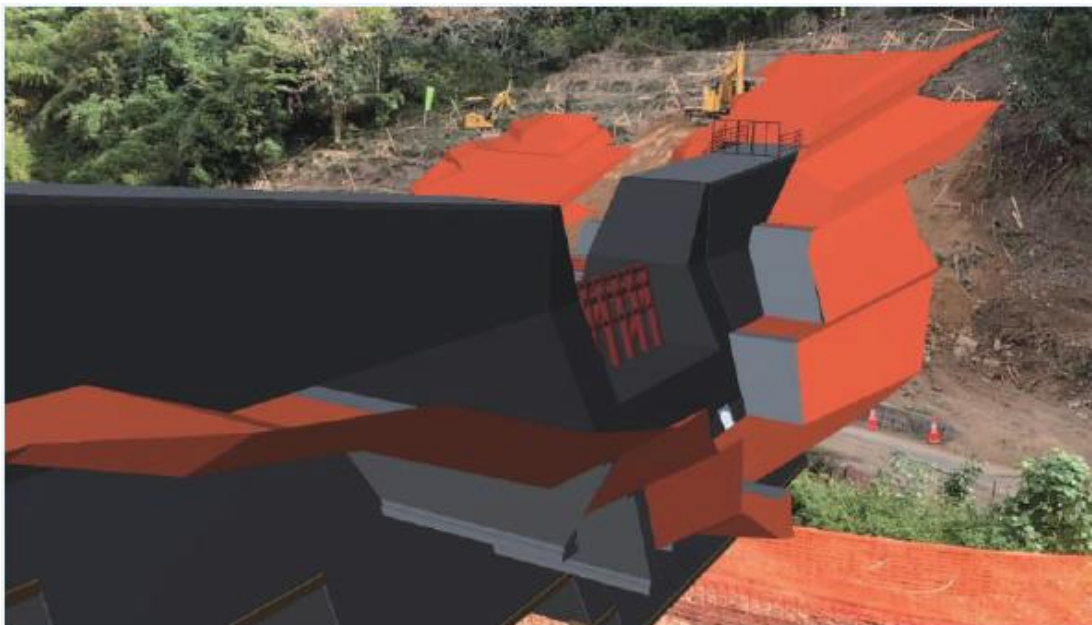
図 5-32 AR 技術を活用した砂防工事の例
