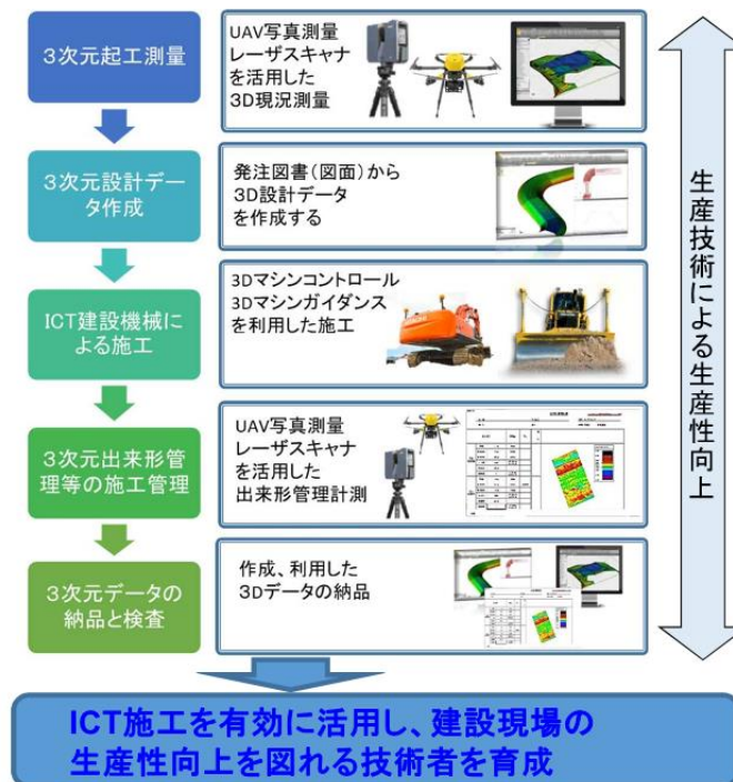
図 5-8 ICT 施工のフレームワーク
