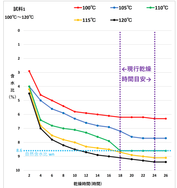
図-3 試料 1: 2～26 時間乾燥: 全温度結果図
