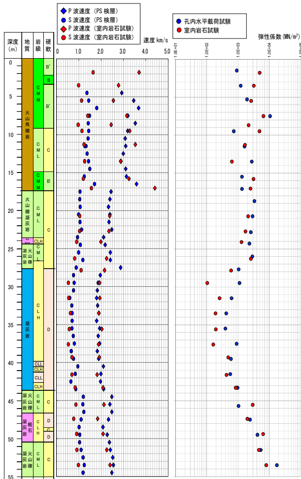
図-4 PS 検層結果と弾性係数及び地質・岩級との比較
