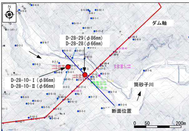
図-1 調査位置平面図
