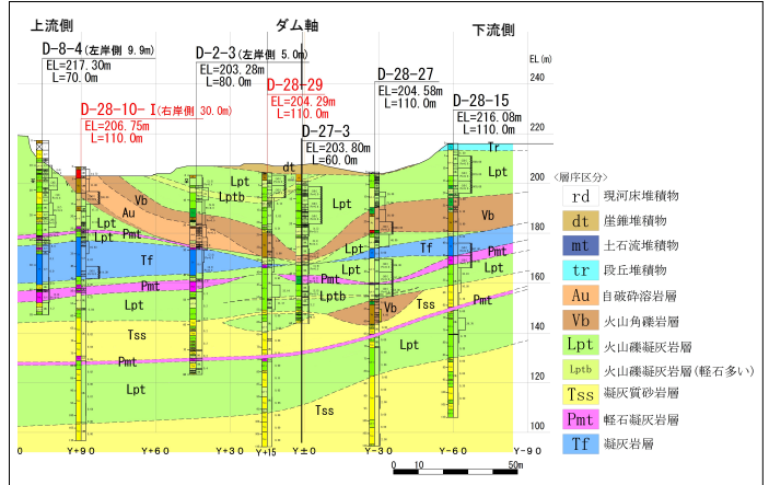
図-2 調査位置地質断面図
