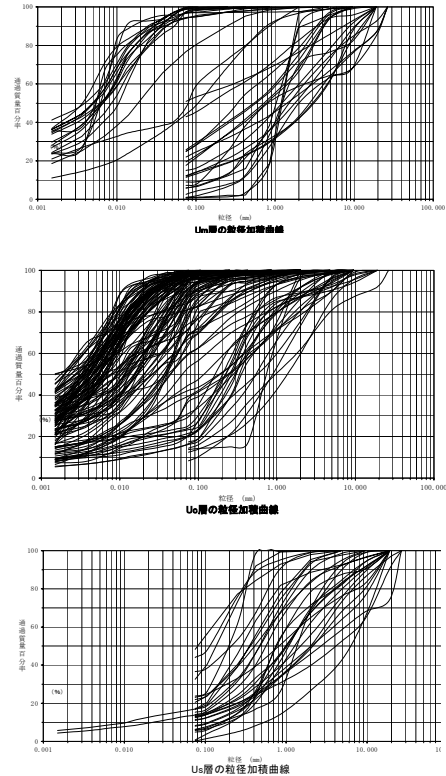
図 - 5 各層の粒径加積曲線 (周南地区)
