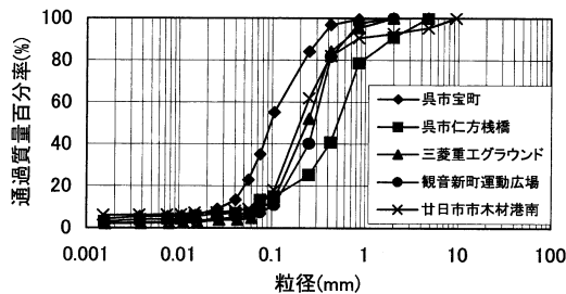
図 - 4 液状化地点の粒径加積曲線 3) (広島地区)
