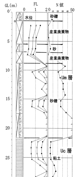
図 - 6 埋立地柱状図
