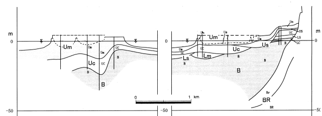
図 - 3 周南地区地質断面図
